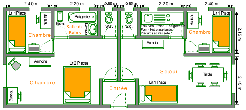
Type E ± 54 m 2
